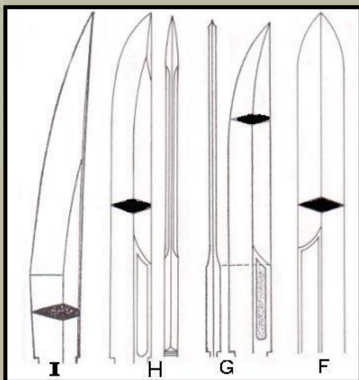
A H és G ábrák az Unokubi zukuri és a Kanmuri otoshi zukuri keresztmetszetek.
